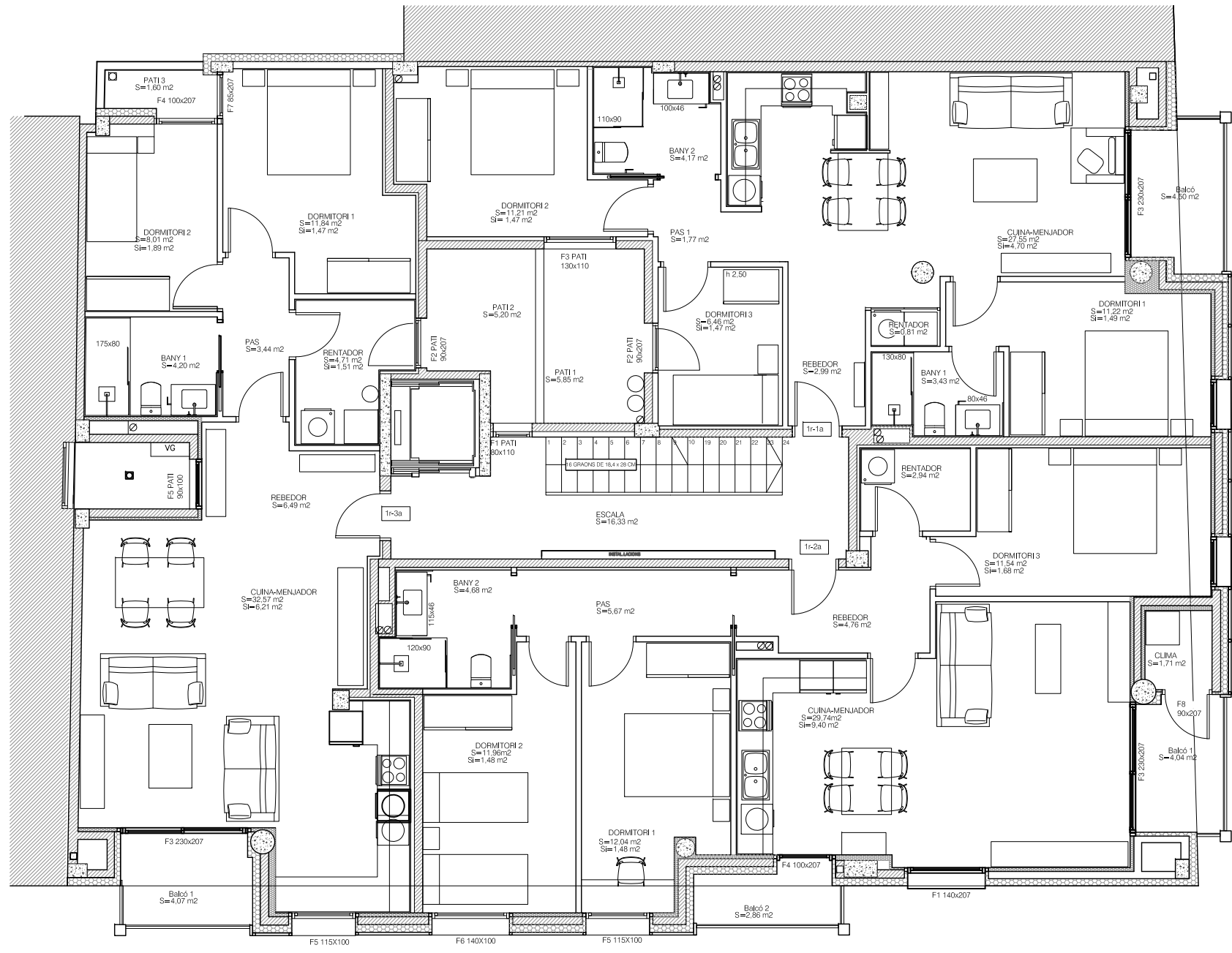
PLANTA PRIMERA
